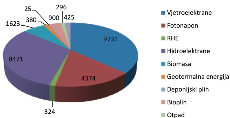
Slika 12: Proizvodnja električne energije po OIE tehnologiji u 2050. godini
