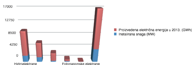
Slika 3: Prikaz proizvodnje električne energije i instalirane snage u 2013. godini unutar RH
