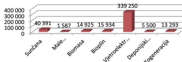
Slika 7: Instalirana snaga po OIE tehnologiji u 2015. godini - elektrane u pogonu
