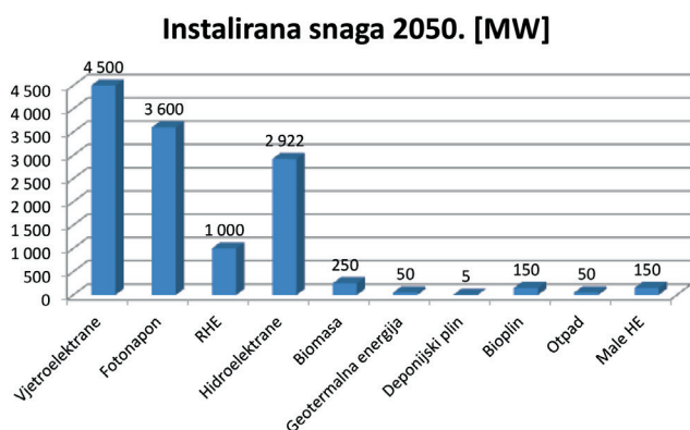
Slika 11: Instalirana snaga po tipu tehnologije 2050. godine
