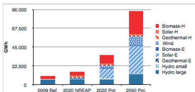
Slika 10: Potencijali obnovljivih izvora energije u Hrvatskoj u 2020. i 2050. godini
